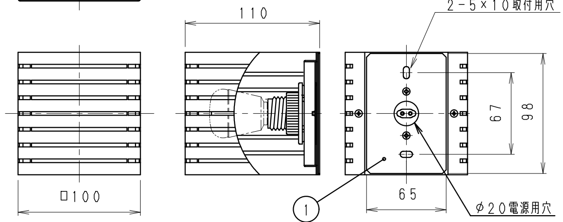
取付寸法図 (A矢視図)
