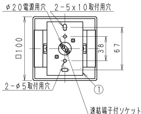
取付面寸法図
