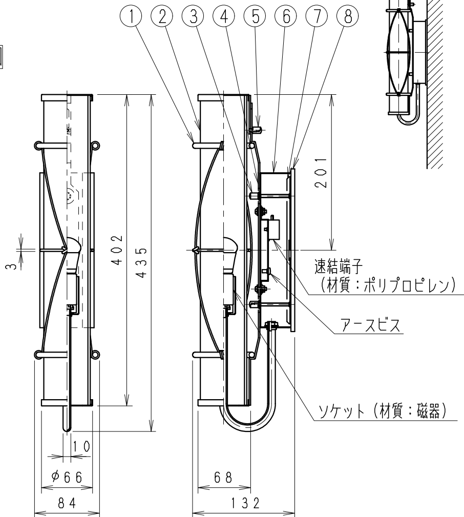
取付面寸法図
