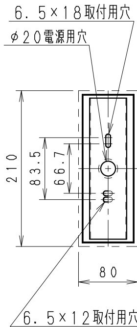
取付面寸法図
