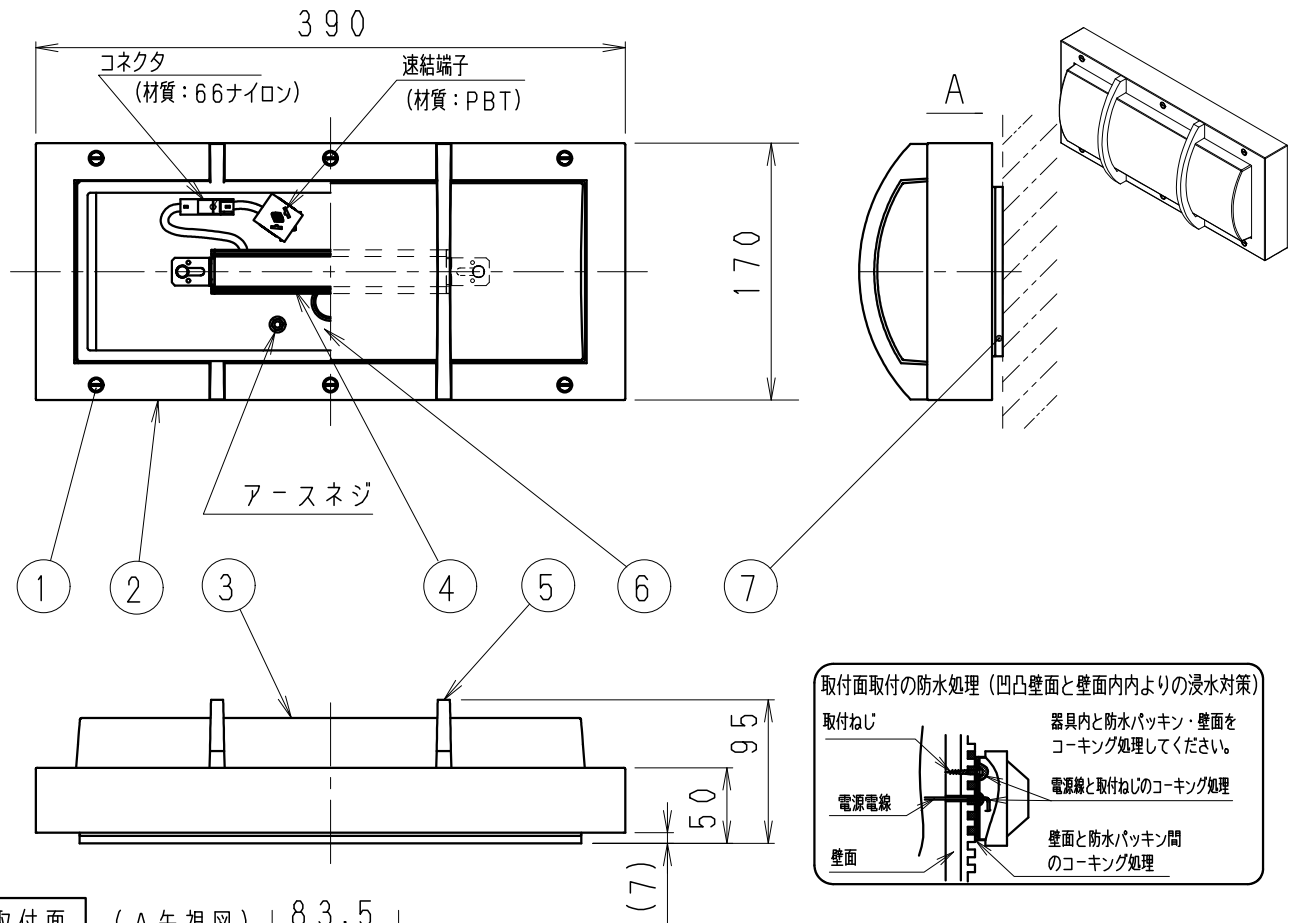
取付面 (A 矢視図)
