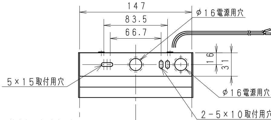
取付寸法図 (A矢視図)
