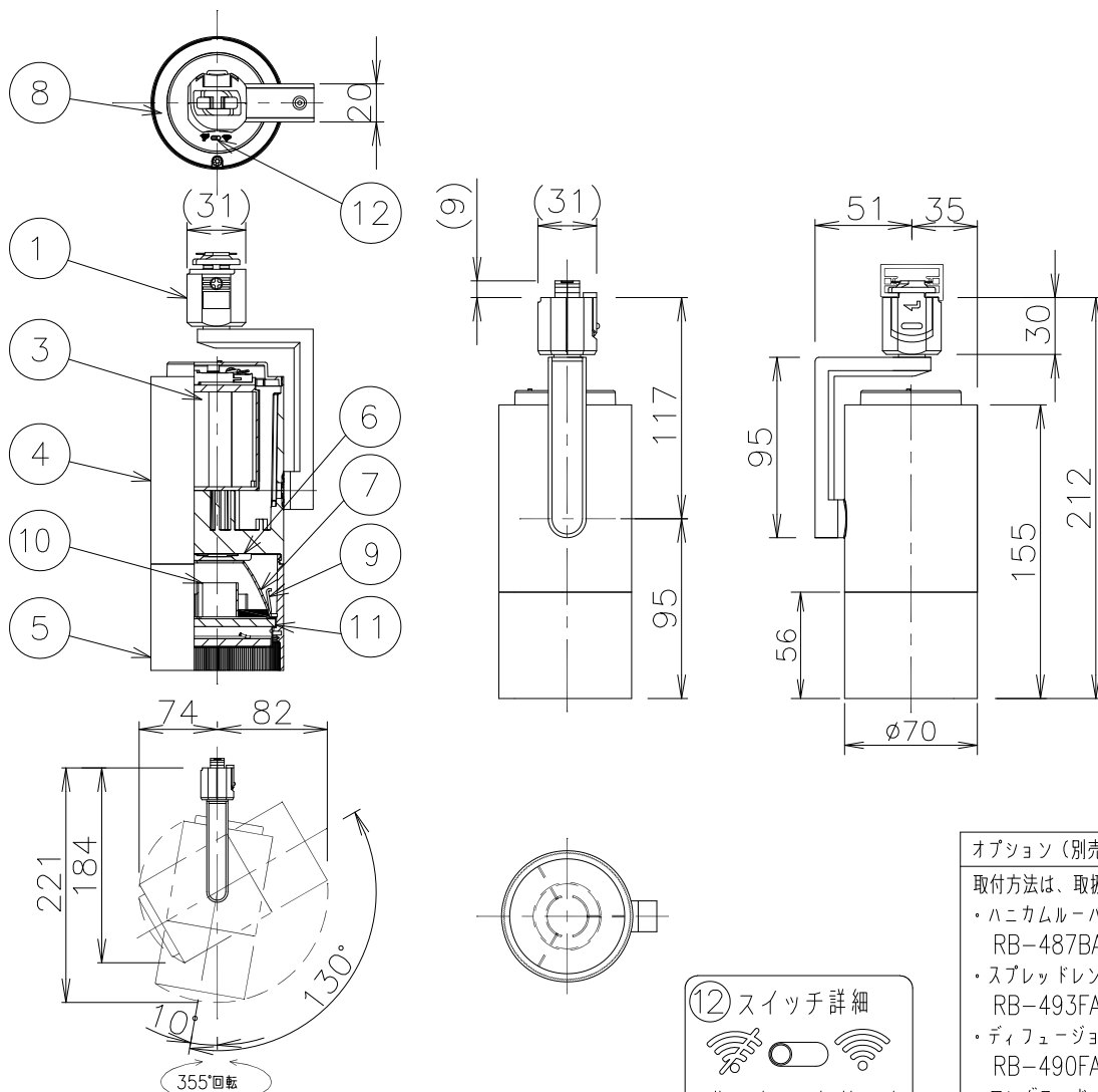
灯具可動範囲図示
