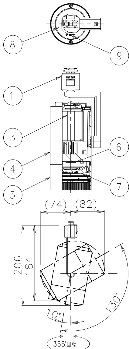
灯具可動範圍図示
