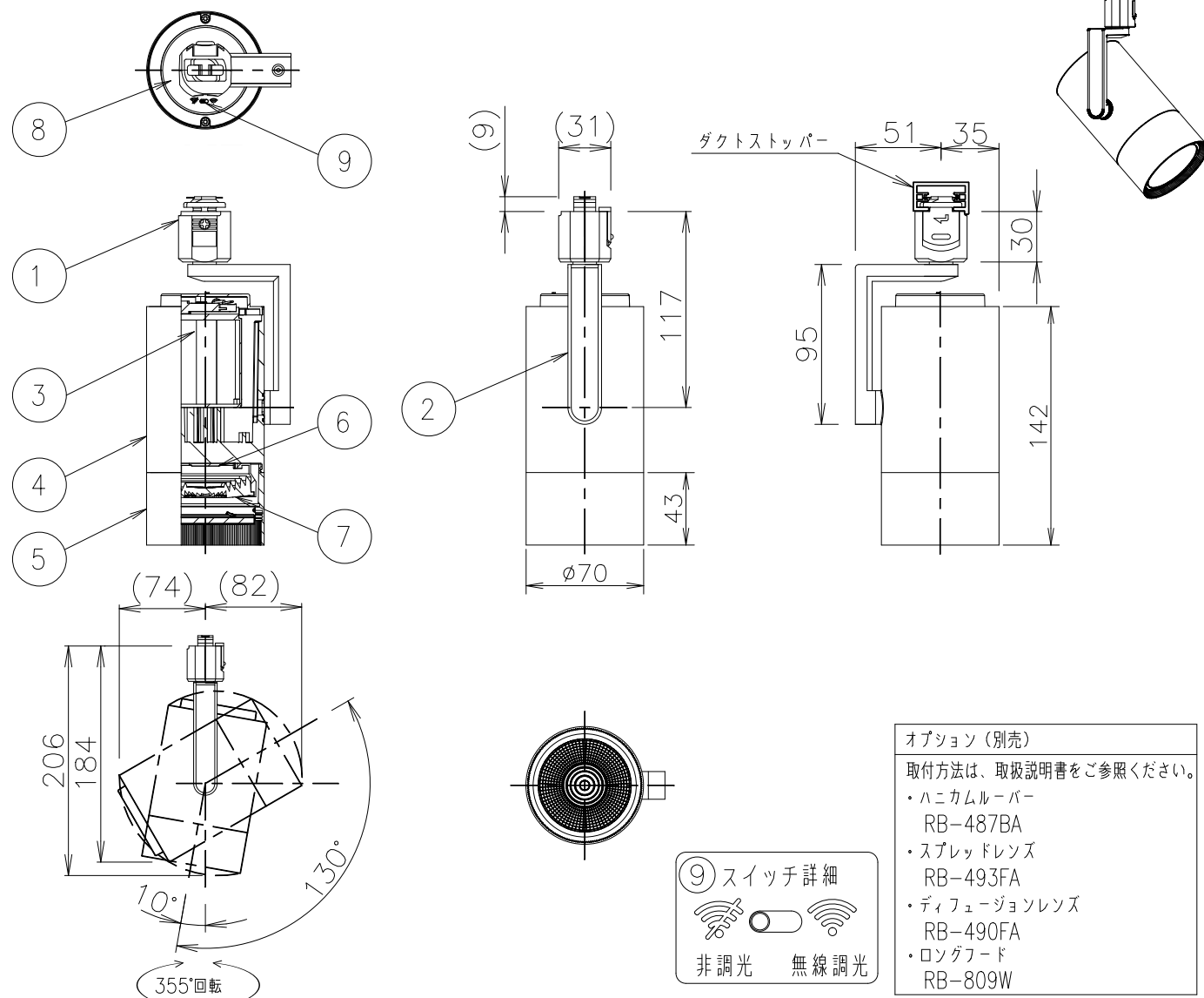
灯具可動範圍図示
