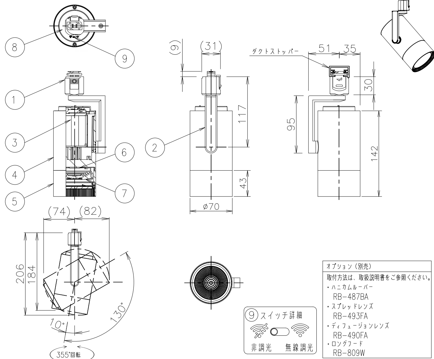
灯具可動範圍圖示
