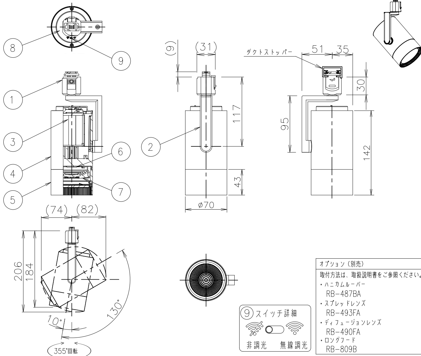
灯具可動範圍図示
