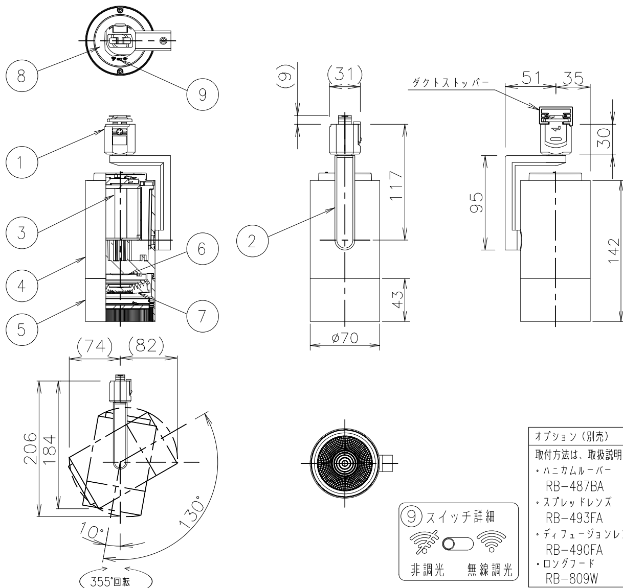
灯具可動範囲図示
