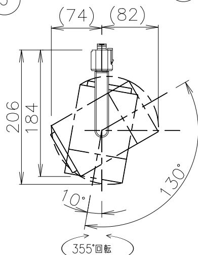
灯具可動範囲図示
