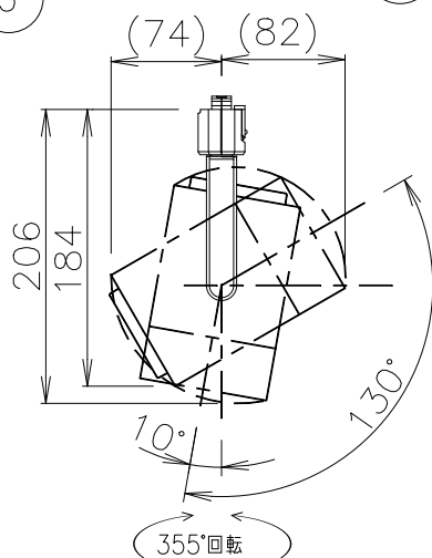
灯具可動範圍図示
