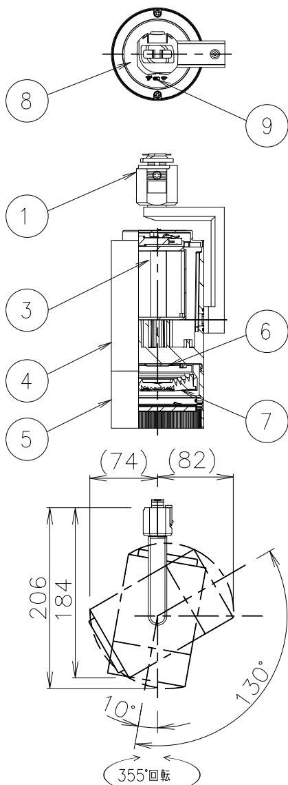
灯具可動範囲図示
