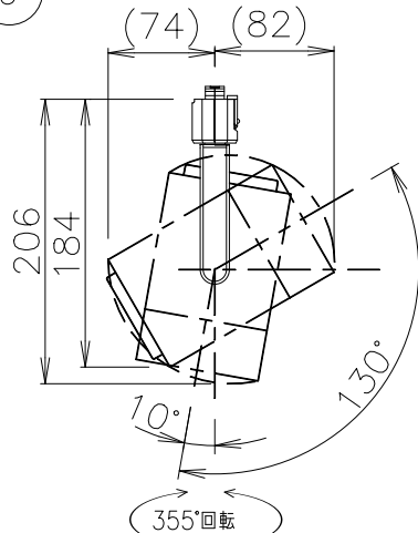
灯具可動範囲図示
