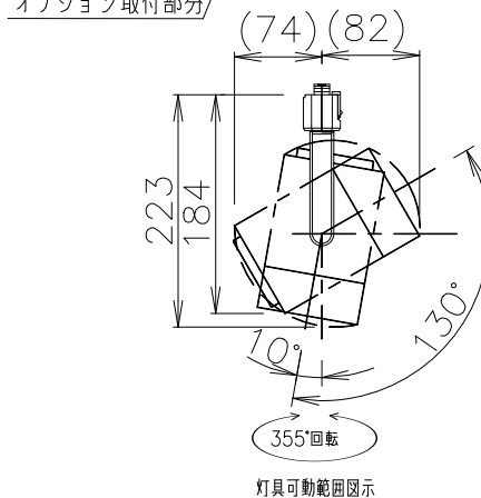
灯具可動範囲図示
