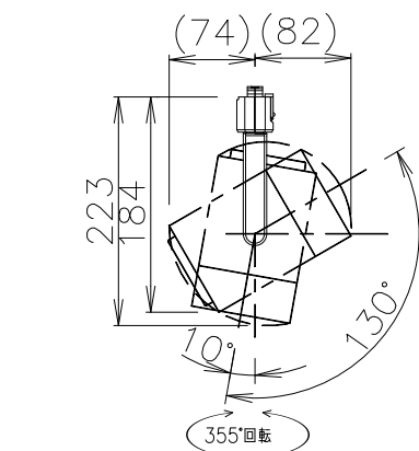
灯具可動範囲図示
