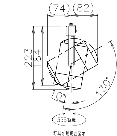
灯具可動範囲図示
