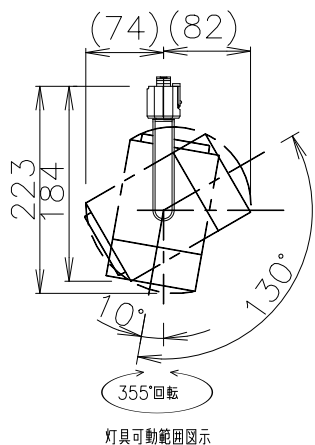
灯具可動範囲図示
