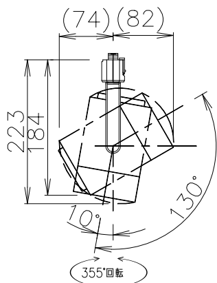
灯具可動範囲図示
