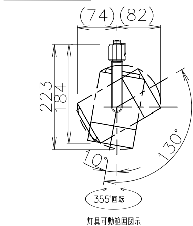
灯具可動範囲図示
