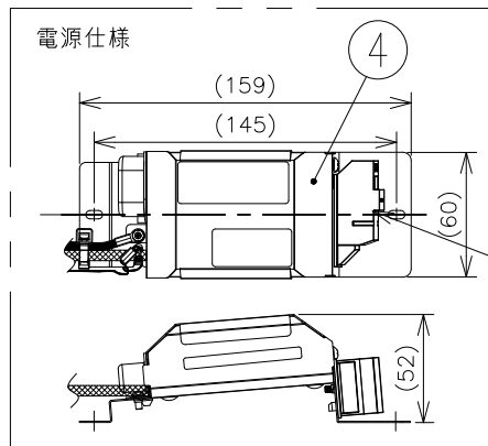
速結送り端子台 (材質: PA) (最大送り容量 4Aまで)
