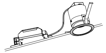
速結送り端子台 (材質: PA) (最大送り容量 4Aまで)
