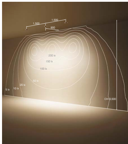
Rs-12ウォールウォッシャー×3灯 使用時配光イメージ
