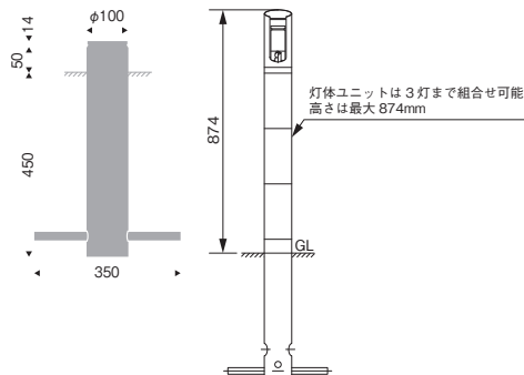
埋込ベースユニット RL-857H ¥14,800 メタリック仕上 (ガンメタリック) 重耐塩塗装 アルミ
