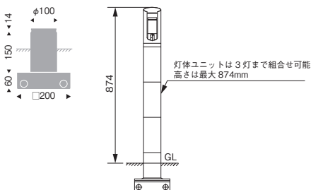
埋込ベースユニット (結線ボックスタイプ) RL-860H ¥21,500 ㊞ メタリック仕上 (ガンメタリック) 重耐塩塗装 アルミ
