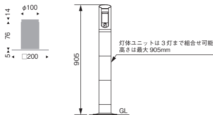
直付ベースユニット RL-858H ¥15,000 ㊞ メタリック仕上 (ガンメタリック) 重耐塩塗装 アルミ
