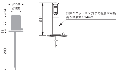
スパイクベースユニット RL-859H ¥13,500 メタリック仕上 (ガンメタリック) 重耐塩塗装 アルミステンレス
