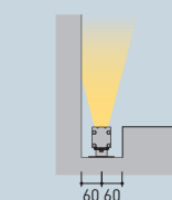
最小施工寸法(単位:mm)
