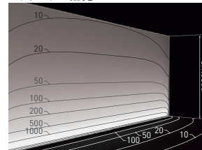
レクタングル配光
