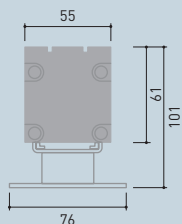
器具サイズ(単位:mm)
