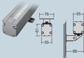
最小施工寸法(単位:mm)
