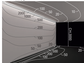
ベース配光
