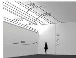
LEDZ リニア 70 拡散配光
