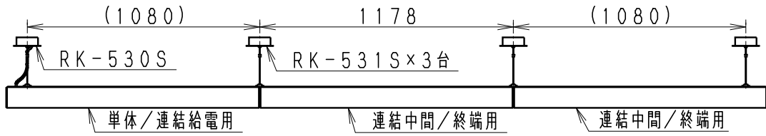
連結取付ピッチ (例) 3台連結時 (S=1/25)
