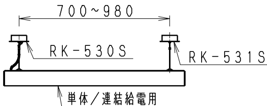
単体取付ピッチ (S=1/25)
