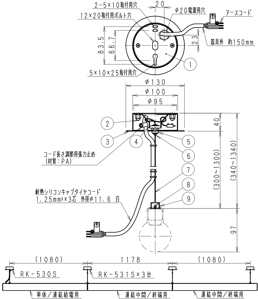
連結取付ピッチ (例) 3台連結時 (S=1/25)
