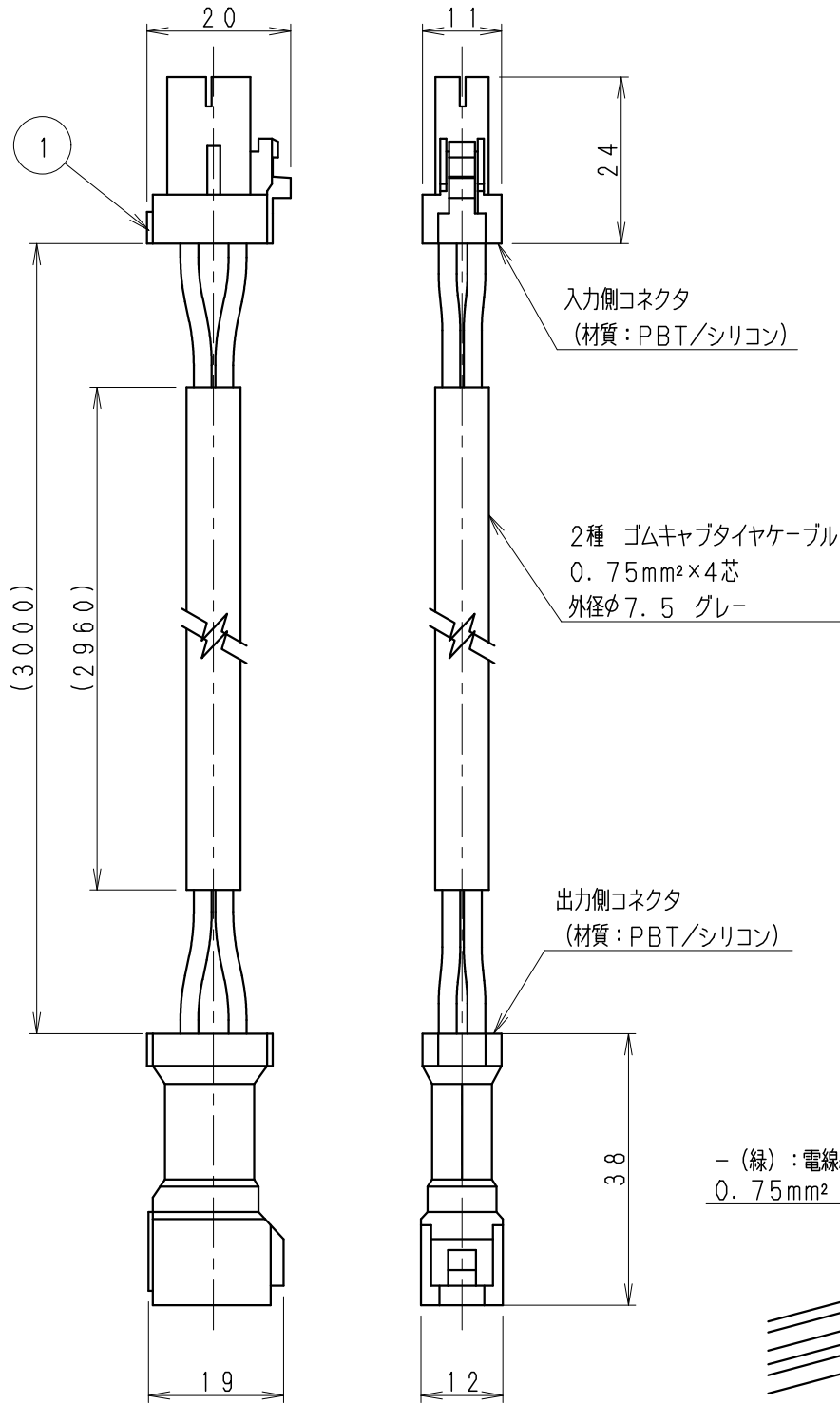
間接照明 Syncaアウトドアリア17 (DC24V)
