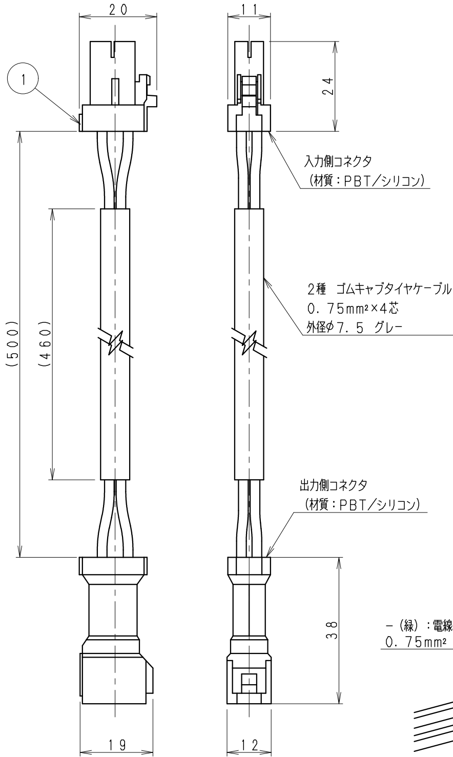
間接照明 Syncaアウトドアリアニア17 (DC24V)
