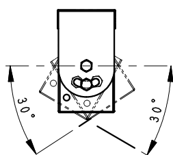
首振り角度
