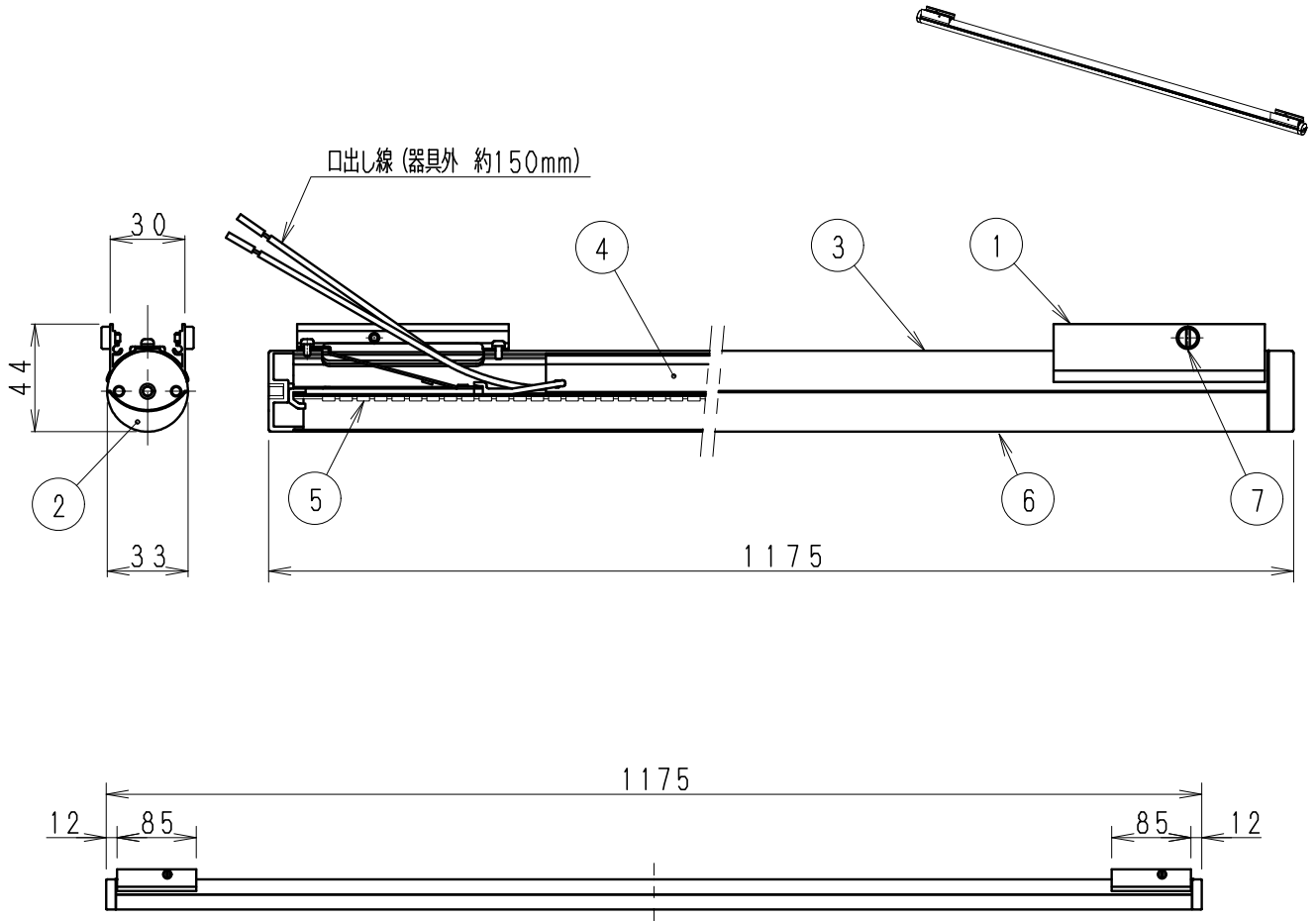
全体図 S = 1/8
