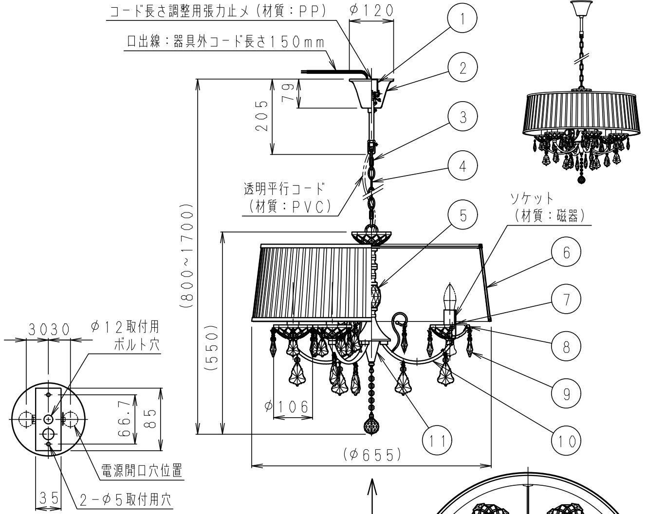
取付面寸法図 S=1/5
