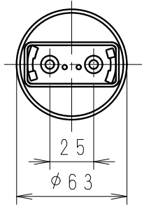
取付面寸法図
