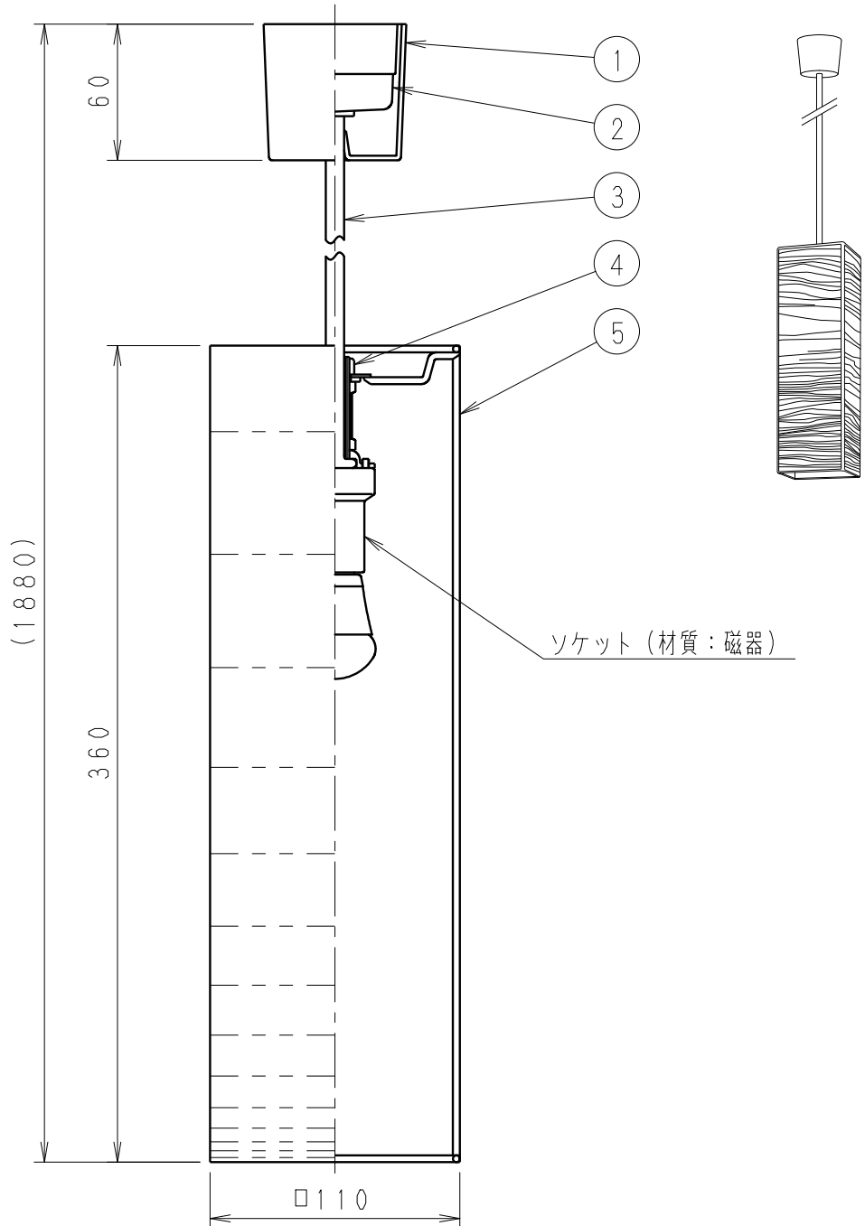
取付面寸法図
