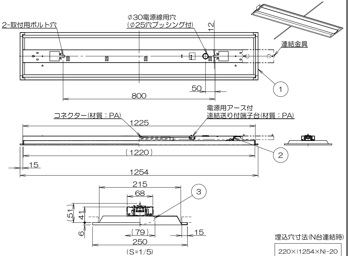
埋込穴寸法
