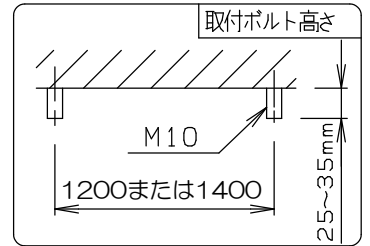
側面図(S=1/3)
