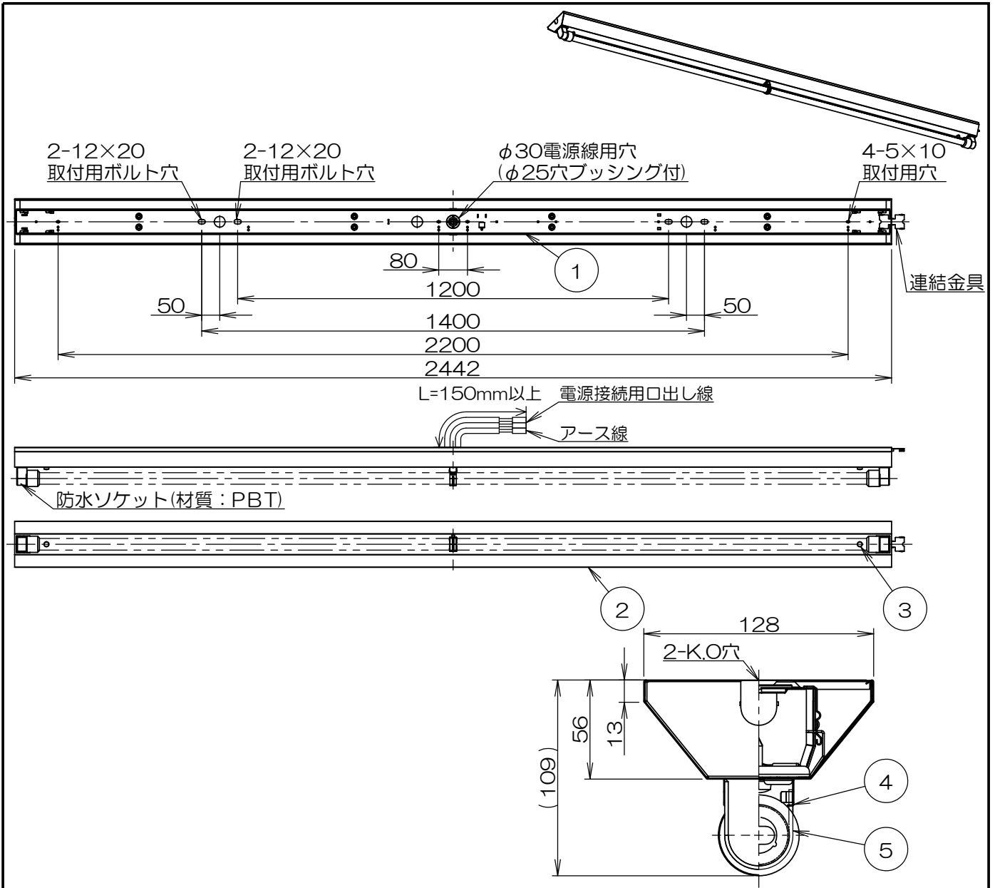
側面図(S=1/3)
