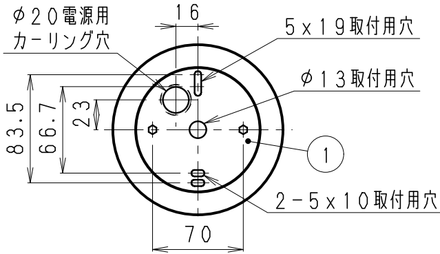
取付面詳細図 S=1/4
