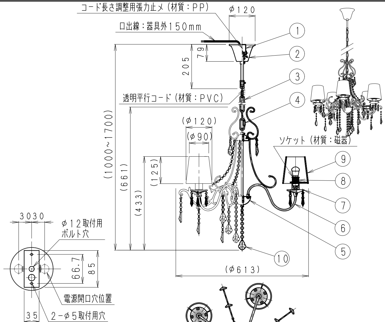
取付面寸法図 S=1/5
