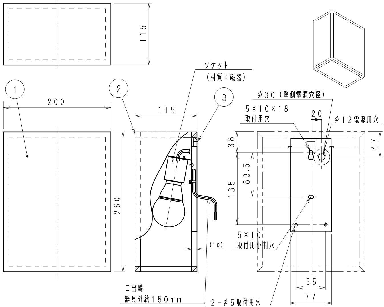
取付け面寸法図 S=1/5
