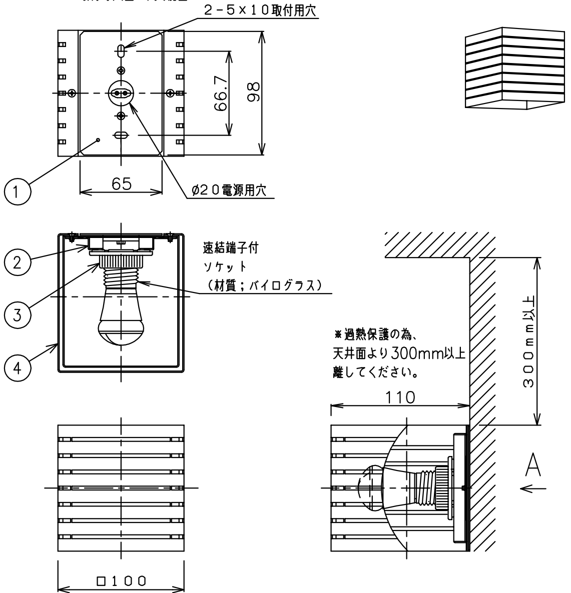
取付寸法図 (A矢视图)
