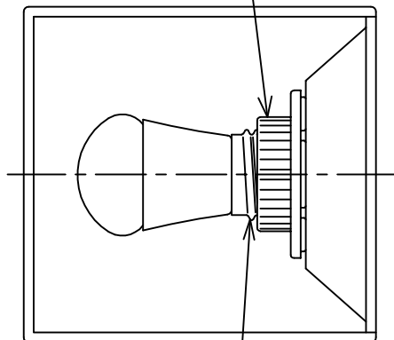
速結式ソケット (材質:パイロガラス)
