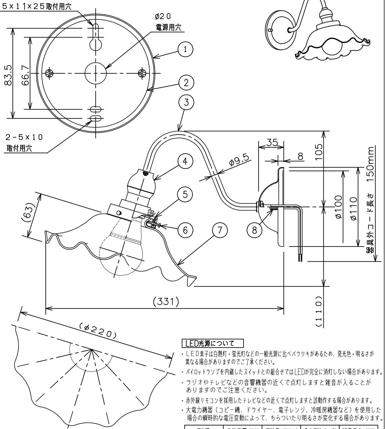
取付面寸法詳細図 (S=1/2)
