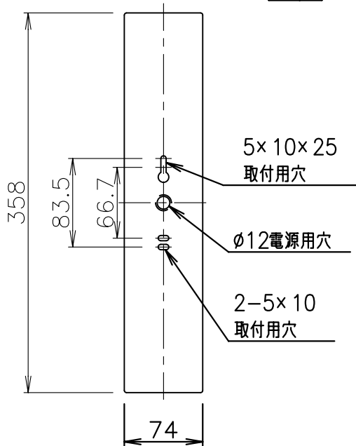
取付面寸法図 S=1/5
