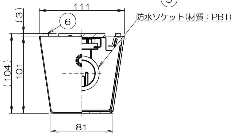
側面図(S=1/3)
