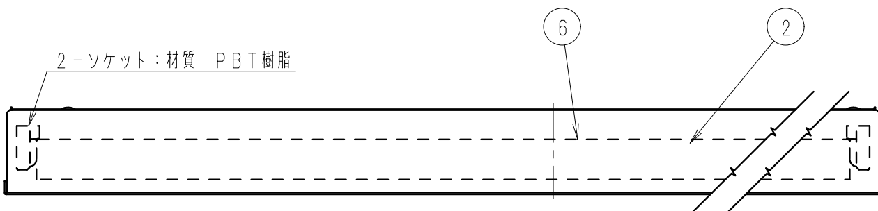
取付寸法図 (A矢視図)
