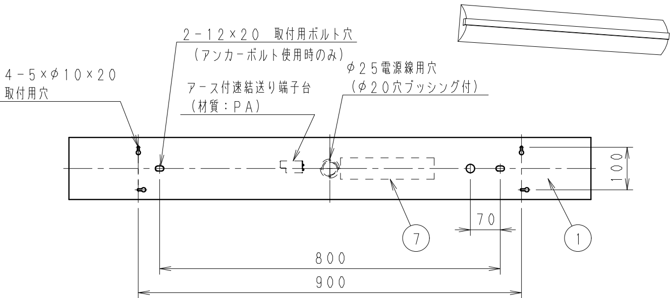
取付寸法図 (A矢視図)
