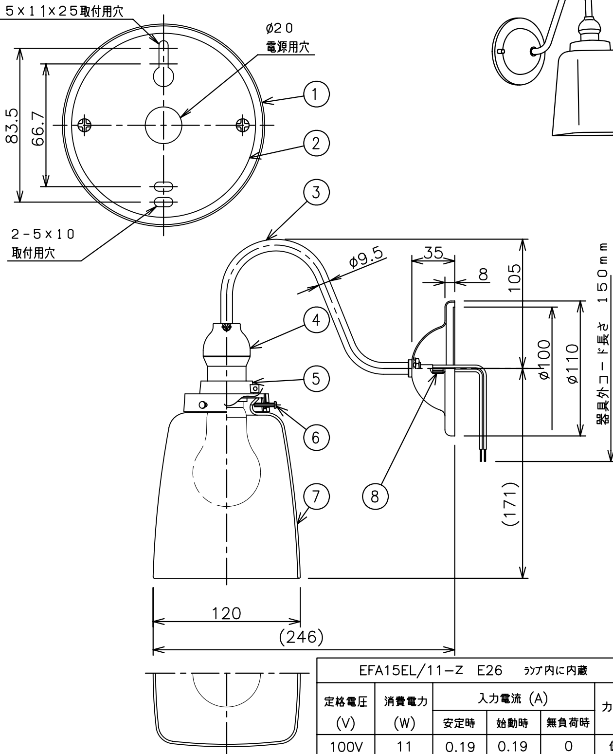
取付面寸法詳細図 (S=1/2)
