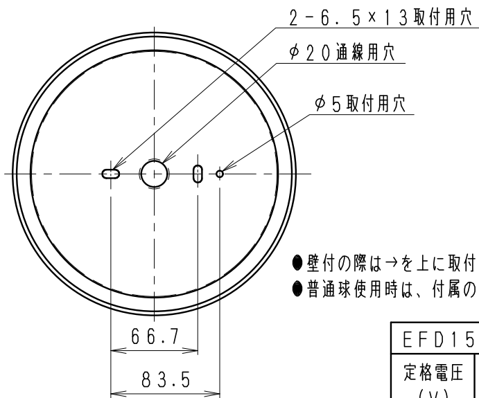
取付面図
