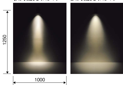
狭角配光(Rs-7)
