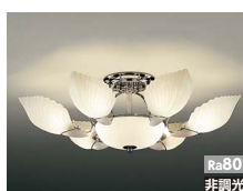
ERC2022S ¥68,000 LEDランプ×8 調 <100V> ● フロストクリプトン球40W形×8相当 消費電力：40.0W 巾(φ811) 高(268)mm 重7.3kg
