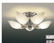
ERC2021S ¥48,500 LEDランプ×5 調 <100V> ● フロストクリプトン球40W形×5相当 消費電力：25.0W 巾(φ660) 高(182)mm 重5.3kg
