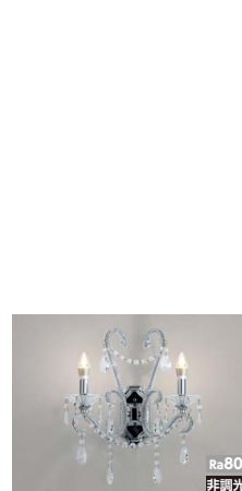
ERB6362S ¥49,800 LEDランプ×2 調 <100V> ● 透明シャンデリア球40W形×2相当 消費電力：10.0W 81.1 lm/W(811 lm) 巾(360) 高(420) 出(184)mm 重1.3kg
